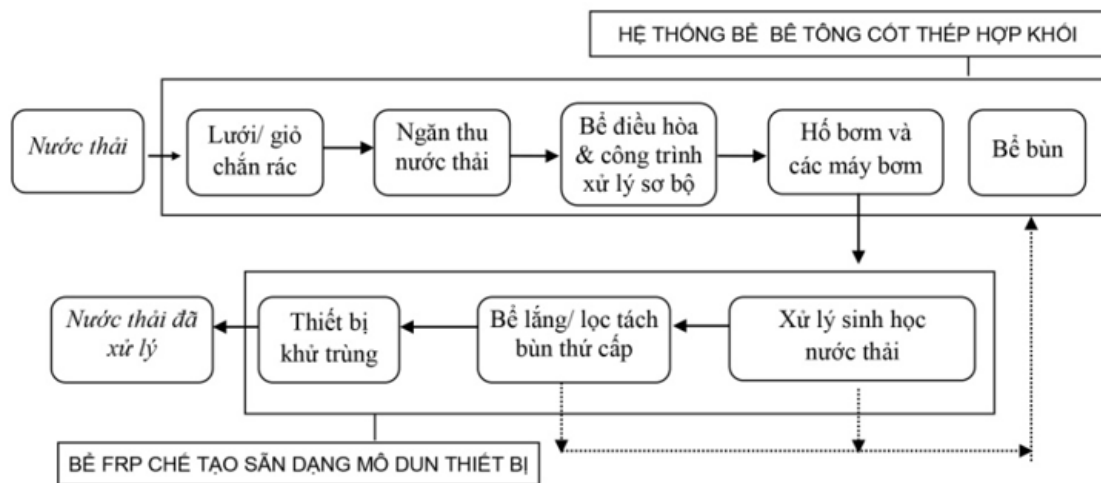
Hình 41. Sơ đồ dây chuyền công nghệ hệ thống XLNT sinh hoạt hợp khối
