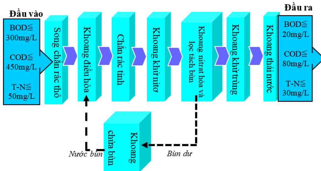
Hình 42. Sơ đồ nguyên tắc hoạt động của hệ thống johkasou
